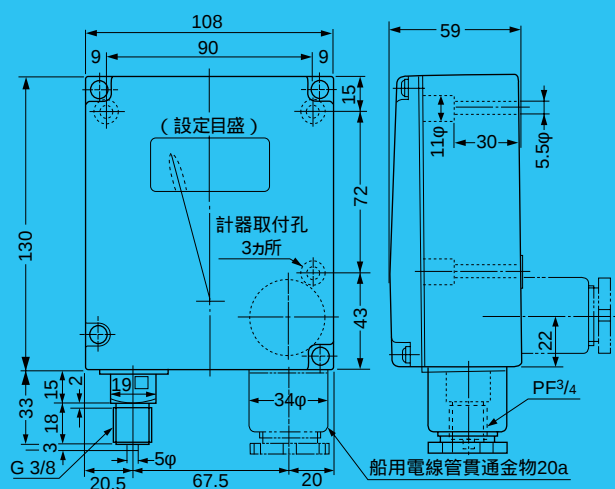
外形寸法図
